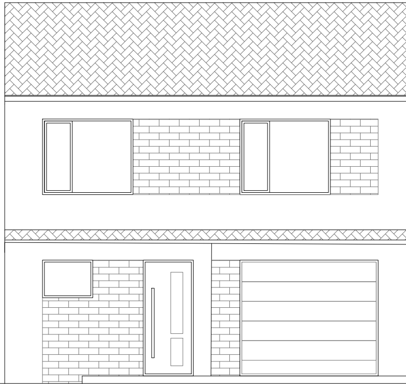
POHLAD ČELNÝ
