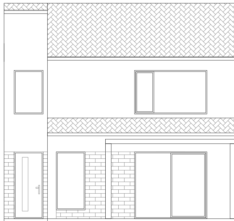
POHLAD ZADNÝ
