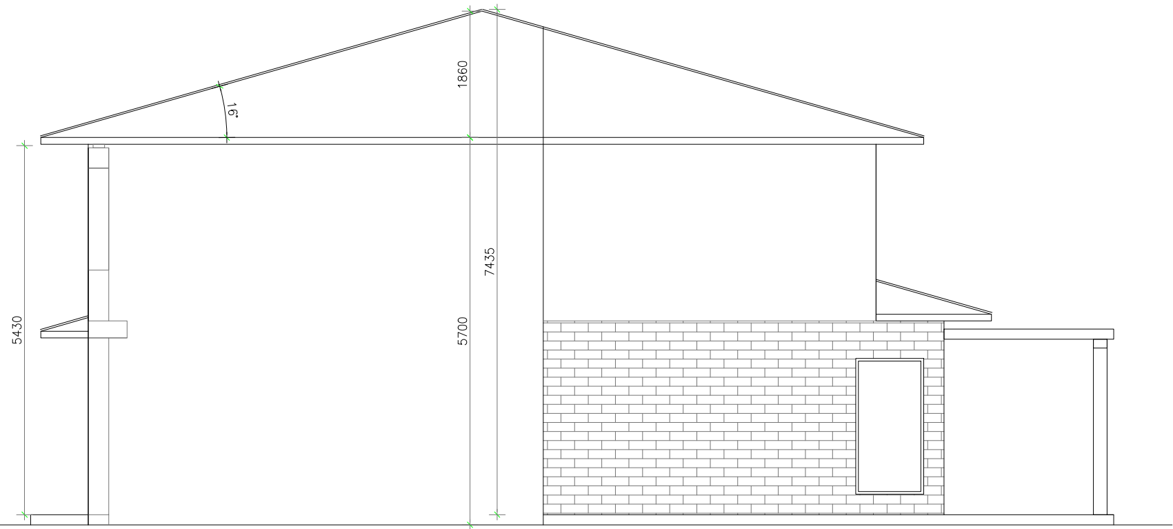
POHLAD BOČNÝ
